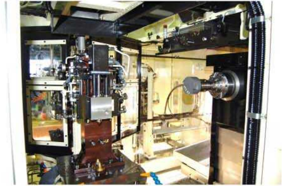
右側マシニングセル、治具部
