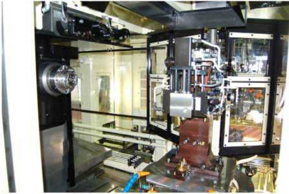
左側マシニングセル、治具部
