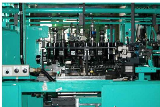
右マシニングセル 工具マガジン
