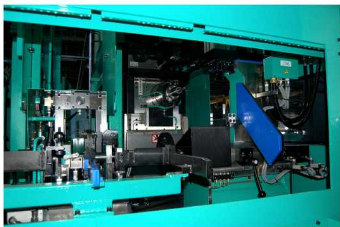
右主軸部、治具部
